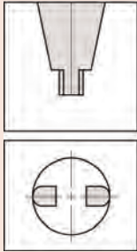
Kerekített mérőfelület a belső mérésekhez
